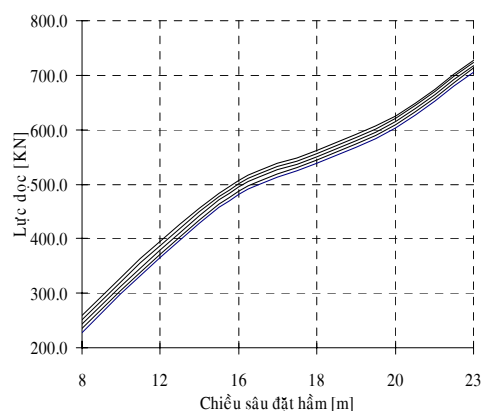
Hình 7. Biểu đồ quan hệ giữa chiều sâu đặt hầm và lực dọc
