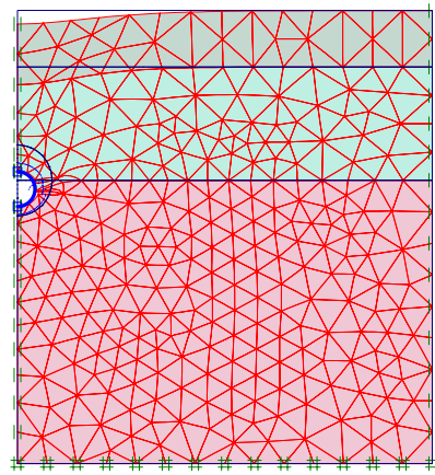
Hình 2. Biểu đồ biến dạng
