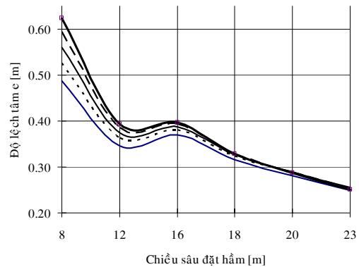
Hình 6. Biểu đồ quan hệ giữa chiều sâu đặt hầm và độ lệch tâm
