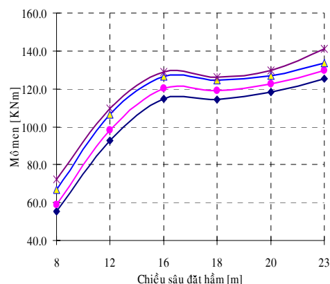
Hình 8. Biểu đồ quan hệ giữa chiều sâu đặt hầm và mômen
