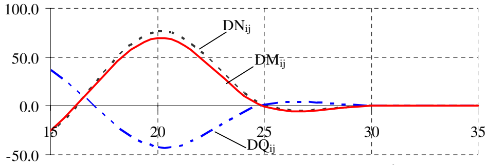
Hình 5 : Quan hệ giữa bán kính ảnh hưởng R và sự thay đổi nội lực
