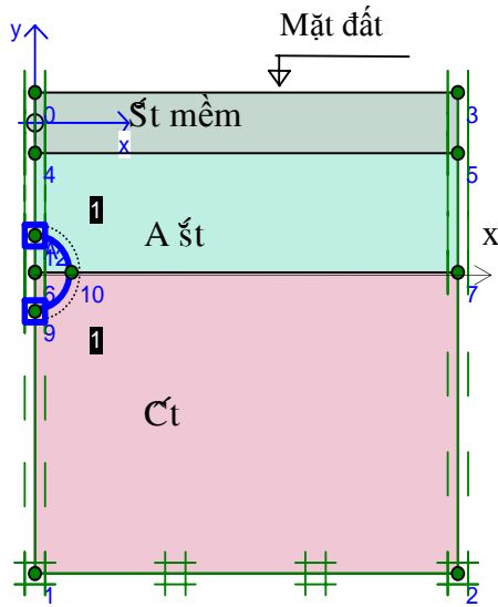
Hình 1. Mô hình bài toán
