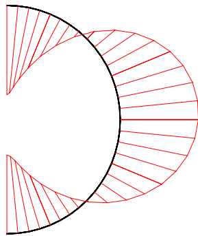
Hình 3. Biểu đồ mômen khi R = 15m
