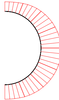
Hình 4. Biểu đồ lực dọc khi R = 15m
