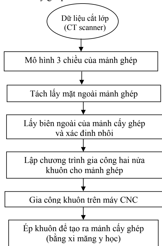
Hình 1: Trình tự chế tạo mảnh cây ghép bằng cách gia công khuôn trên máy phay CNC
