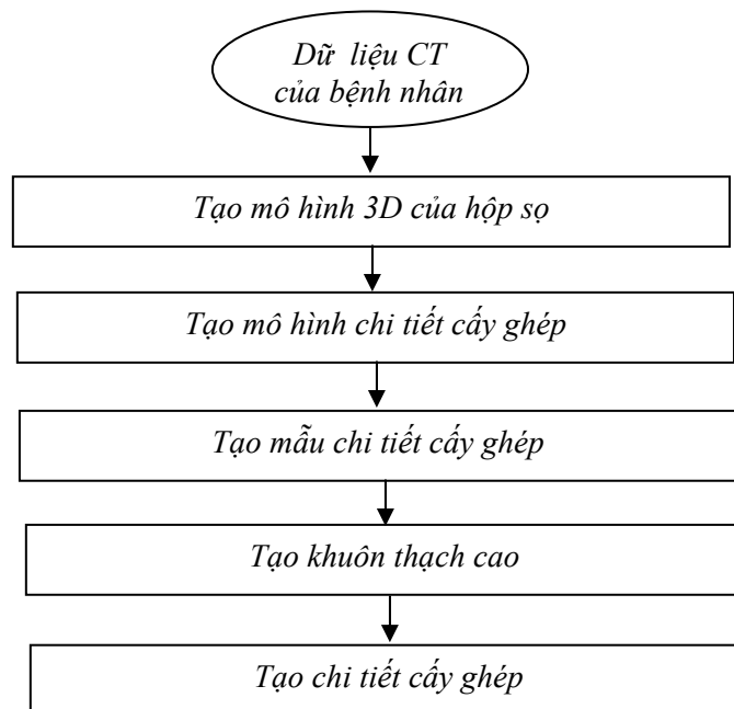
Hình 3 : Tổng thể của qui trình chế tạo chi tiết cấy ghép bằng công nghệ tạo mẫu nhanh
