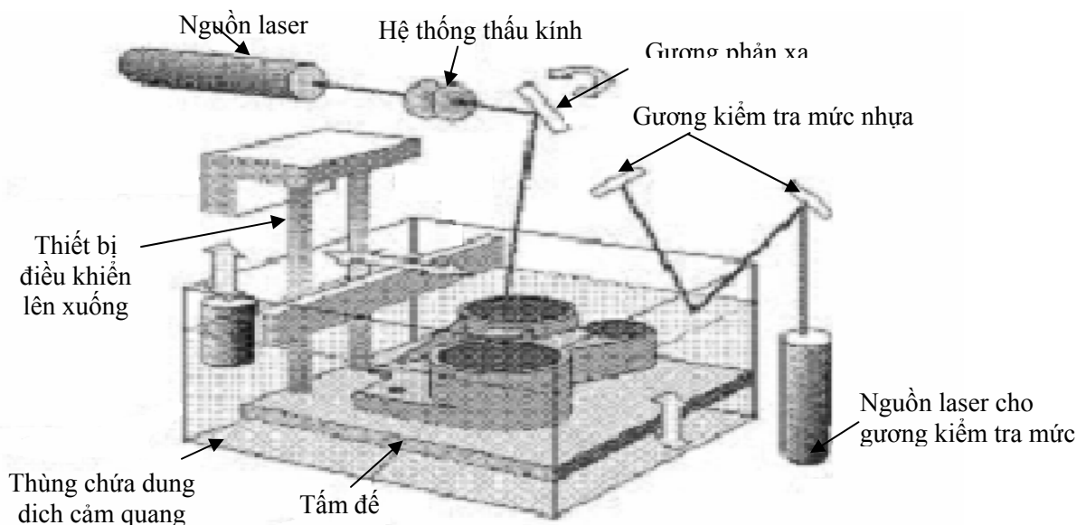
Hình 2 : Sơ đồ nguyên lý hoạt động của SLA
